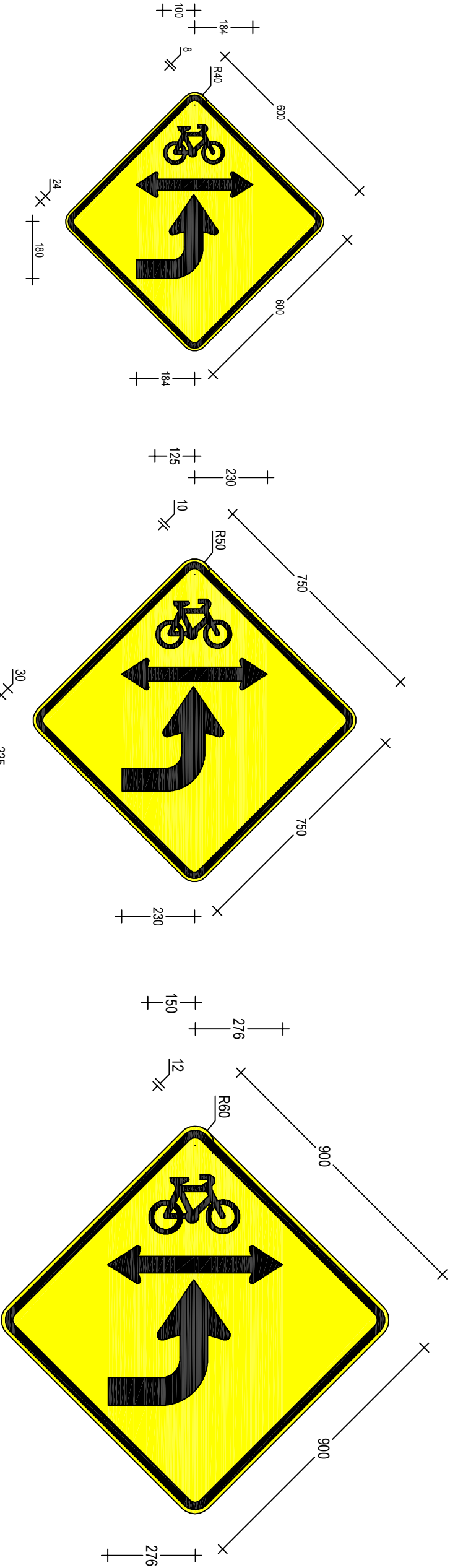
W8-200n(A) 600 x 600
